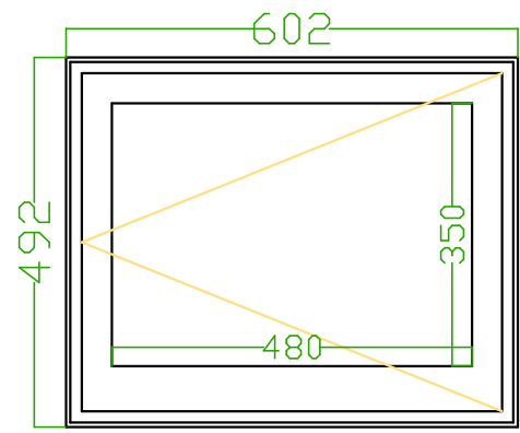
Eco 600 met modern inbouwkader
