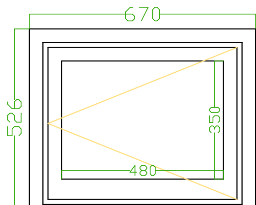
Eco 600 met 3-zijdig klassiek kader
