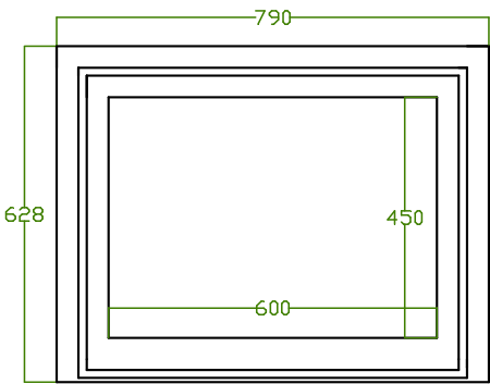
Variant 720 + 3-zijdig klassiek kader
