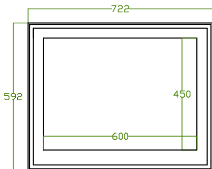
Variant 720 + modern inbouwkader
